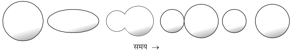
चित्र 27.2: द्रव-बूंद मॉडल के अनुसार किसी नाभिक का विखंडन
