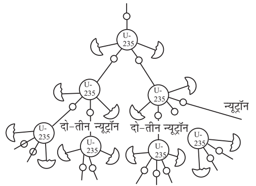
चित्र 27.4 : नाभिकीय शृंखला अभिक्रिया
