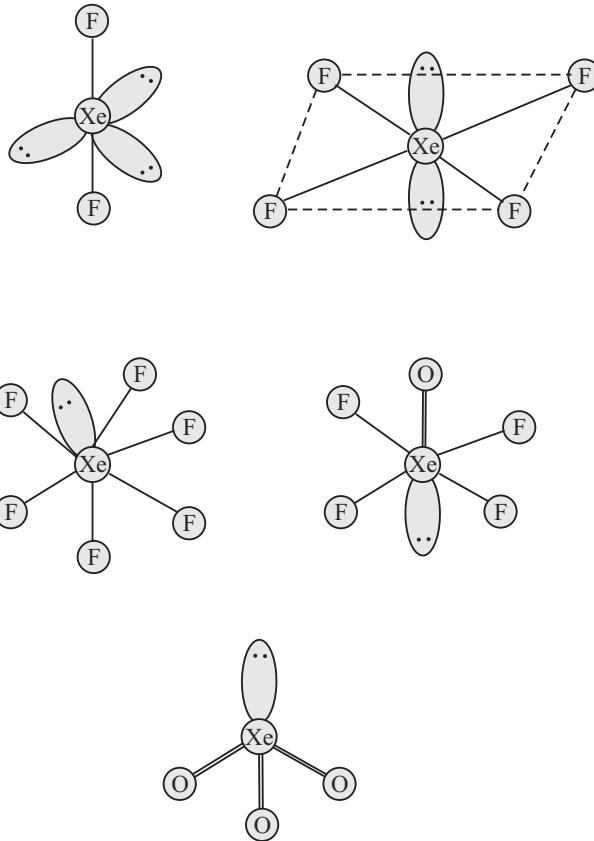
चित्र 20.3 : \text{XeF}_2 , \text{XeF}_4 , \text{XeF}_6 , \text{XeO}_3 और \text{XeOF}_4 की संरचनाएँ
