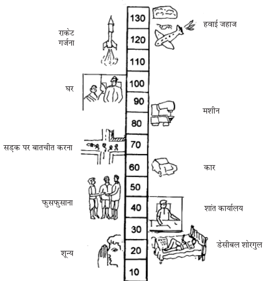
चित्र 27.6 ध्वनि प्रदूषण के स्रोत
