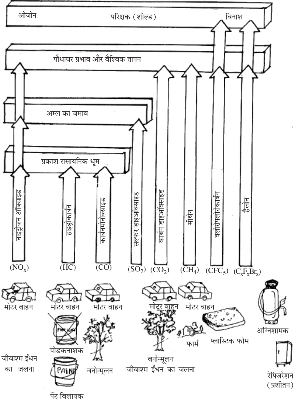
चित्र 27.1 वायु प्रदूषण के मुख्य प्रभाव
